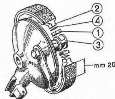
Fig. 15 - Recupero del giuoco dovuto al consumo delle guarnizioni dei freni.
