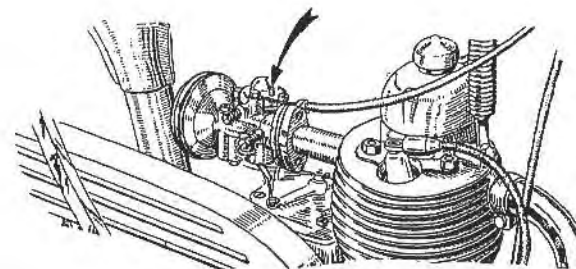
Fig. 4 - Agitatore del galleggiante sul carburatore « Weber ».
