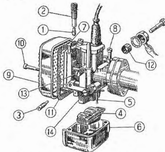
Fig. 18 - Pulizia carburatore « Dell'Orto ».
