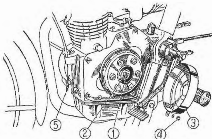
Fig. 12 - Regolazione giuoco comando frizione.
