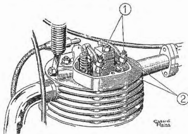
Fig. 10 - Regolazione giuoco comando valvole
