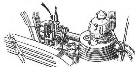
Fig. 4 - Agitatore del galleggiante sul carburatore « Dell'Orto ».
