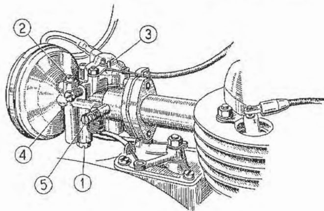
Fig. 8 - Carburatore « Weber »
