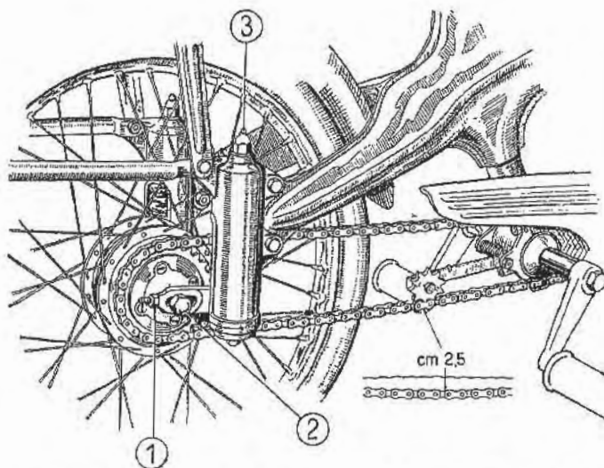
Fig. 14 - Regolazione tensione catena - Sospensione posteriore.
