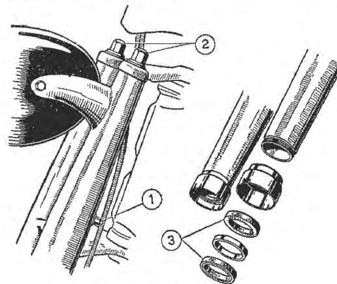
Fig. 7 - Forcella telescopica.
