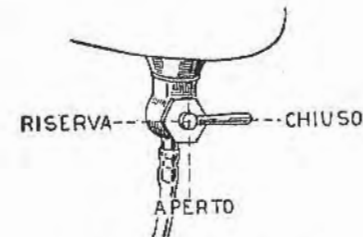
Fig. 1 - Rubinetto benzina.
