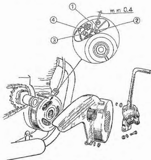
Fig. 11 - Regolazione contatti del ruttore.
