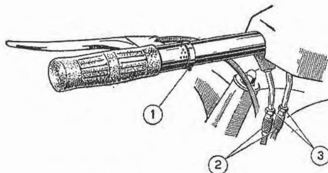
Fig. 13 - Regolazione comando cambio.
