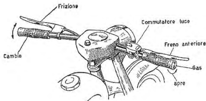
Fig. 2 - Manubrio e comandi.
