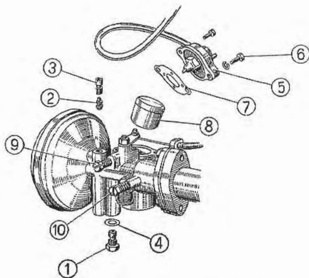
Fig. 17 - Pulizia carburatore « Weber ».
