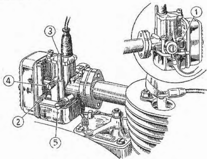
Fig. 9 - Carburatore « Dell'Orto ».
