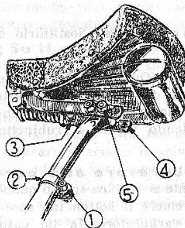
Fig. 8 - Regolazione della sella
