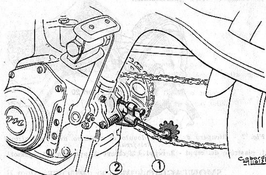
Fig. 6 - Regolazione della tensione della catena di trasmissione
