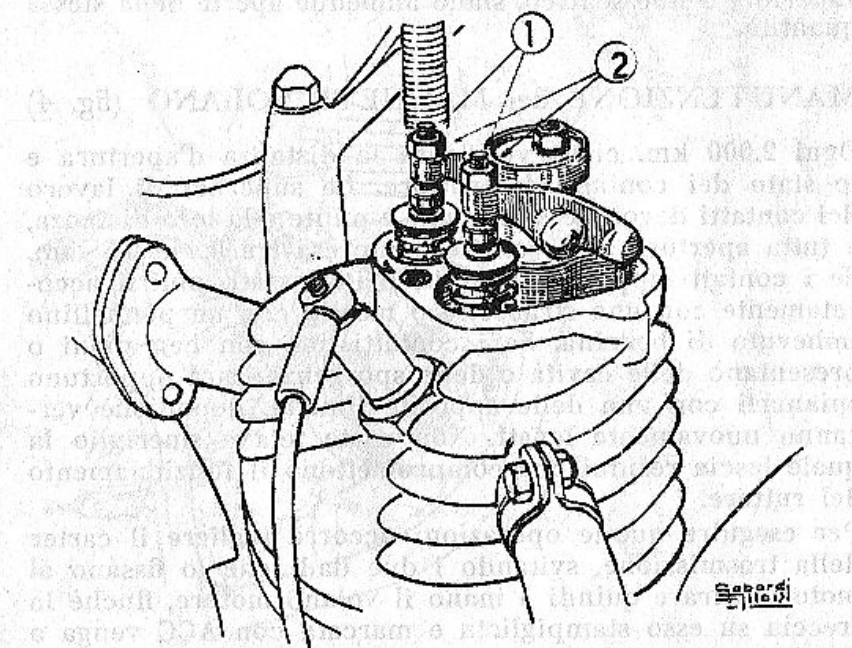
Fig. 3 - Regolazione del giuoco del comando delle valvole
