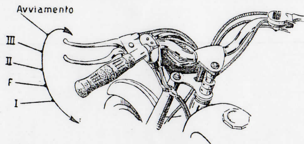
Fig. 5 - Posizioni della manopola comando cambio.
