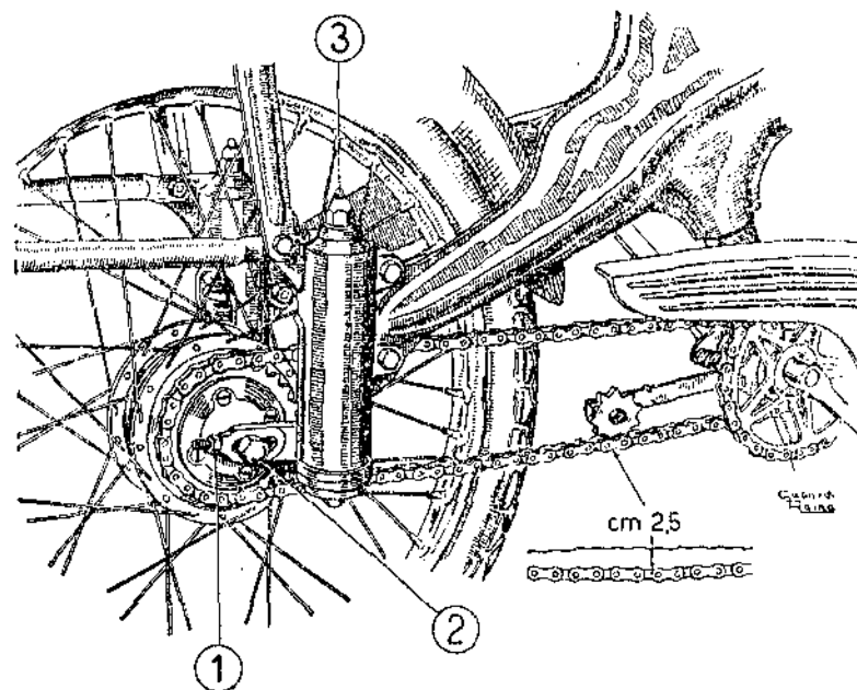
Fig. 12 - Regolazione tensione catena - Sospensione posteriore
