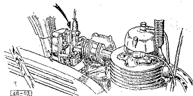
Fig. 3 - Agitatore del galleggiante sul carburatore « Dell'Orto »
