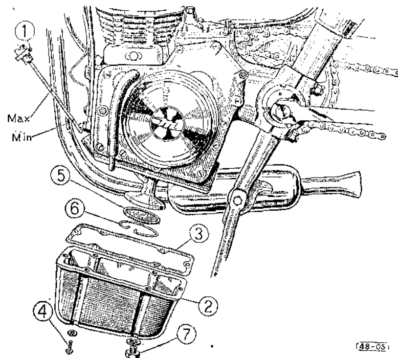
Fig. 5 - Astina controllo livello olio - Coppia smontata per ricambio dell'olio e pulizia del filtro
